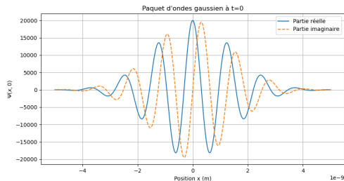
Parties réelle et imaginaire à t = 0 (partie 2).
